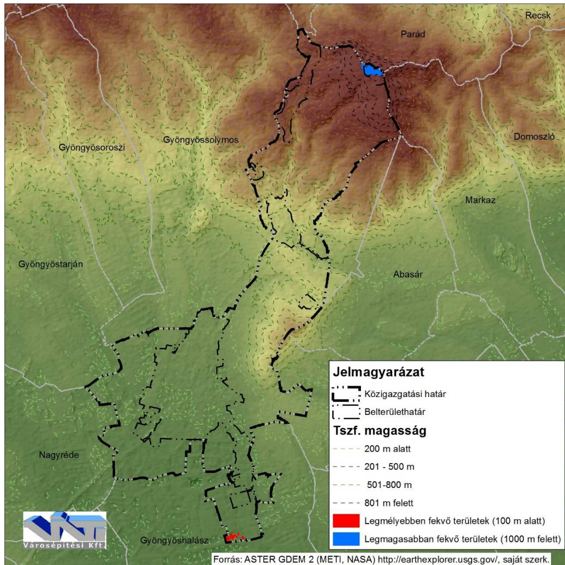
3. ábra Gyöngyös domborzati viszonyai (Forrás: ASTER GDEM 2 (METI, NASA) http://earthexplorer.usgs.gov/ , szerk. VÁTI Városépítési Kft.)
