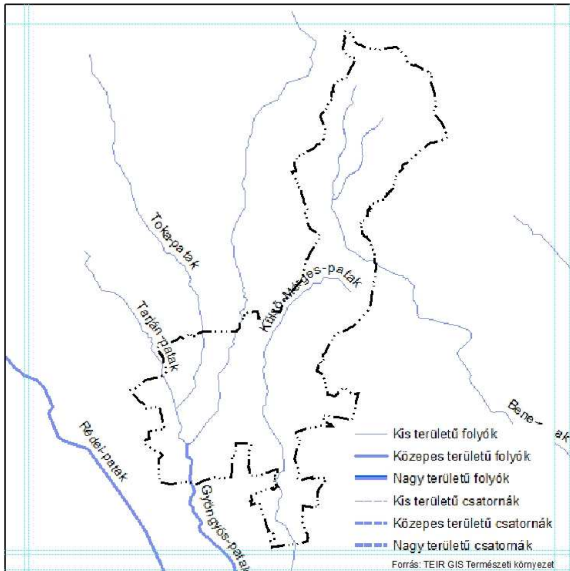
4. ábra Főbb vízfolyások Gyöngyös területén (Forrás: TEIR GIS Természeti környezet)
